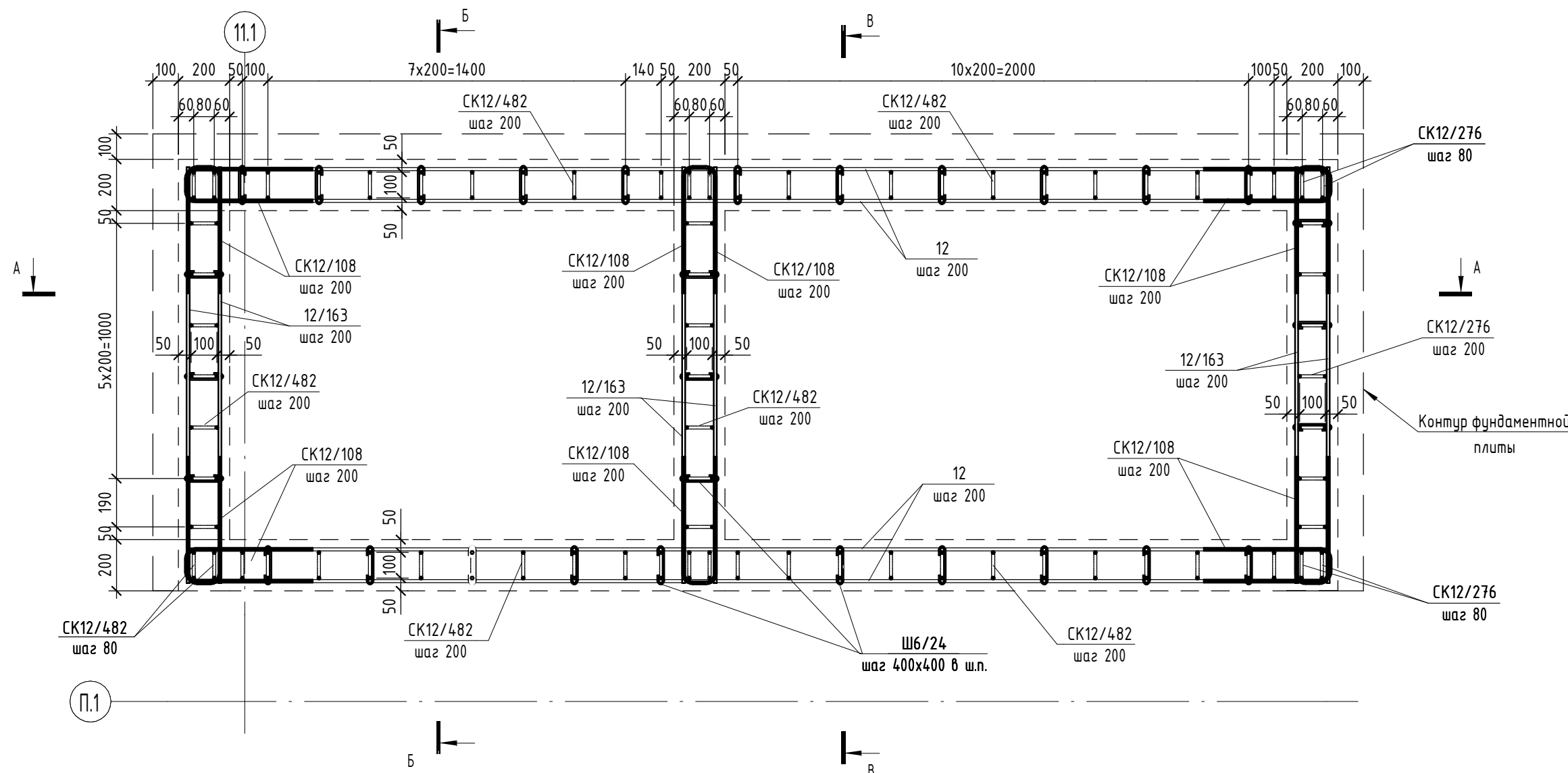
Схема армирования стен входной группы в/о 11.1/П.1 на отм -1,700
