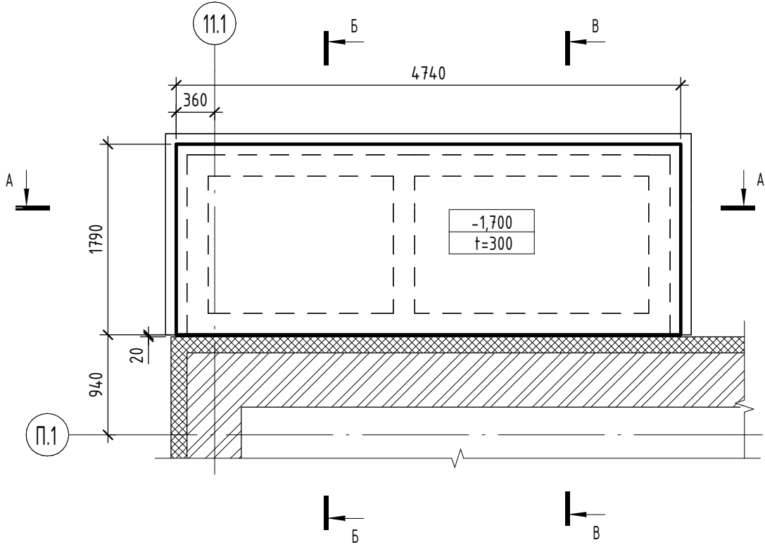
Схема расположения фундаментной плиты входной группы в/о 11.1/П.1 на отм. -1,700
