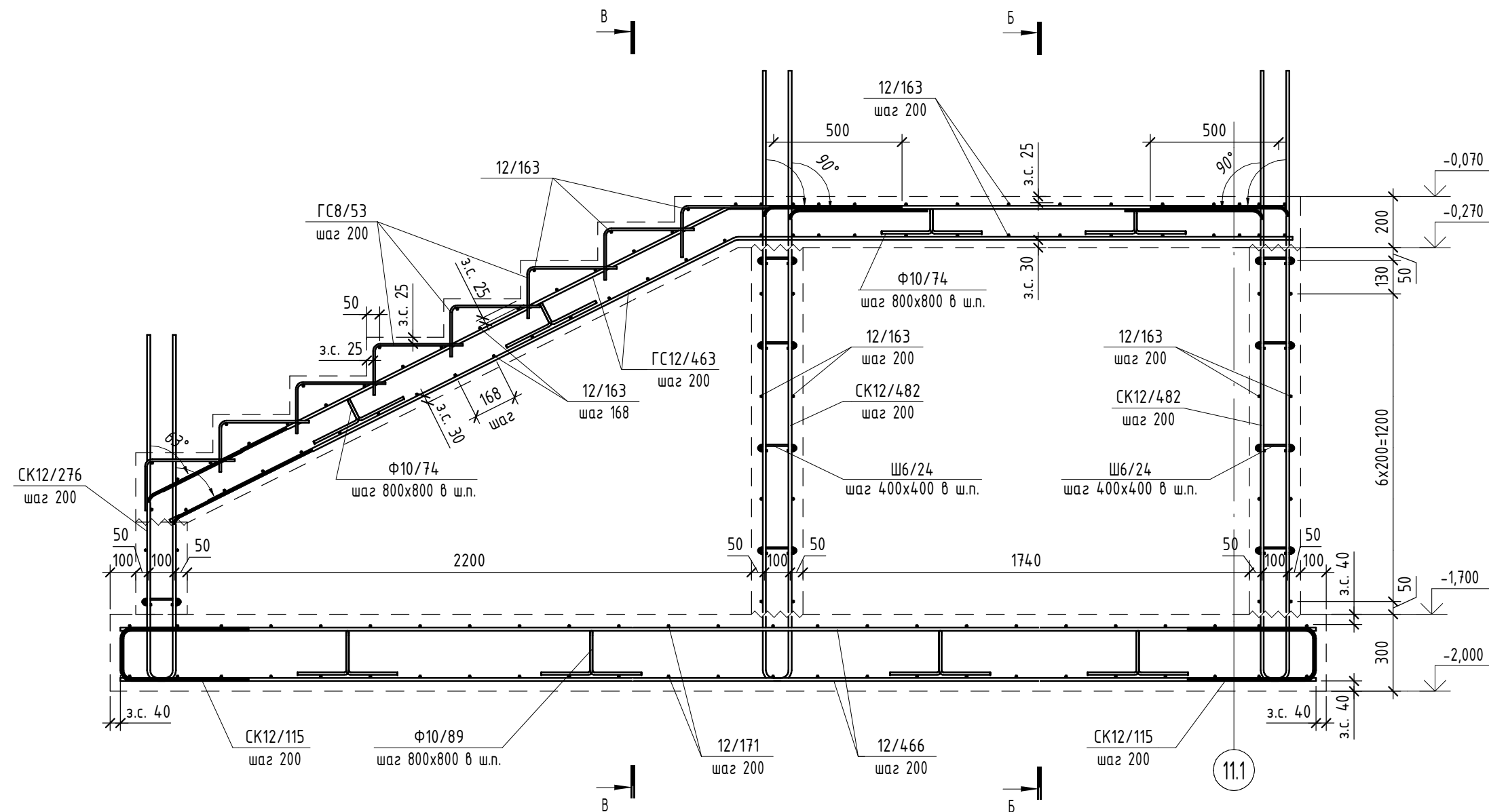
А-А Армирование
